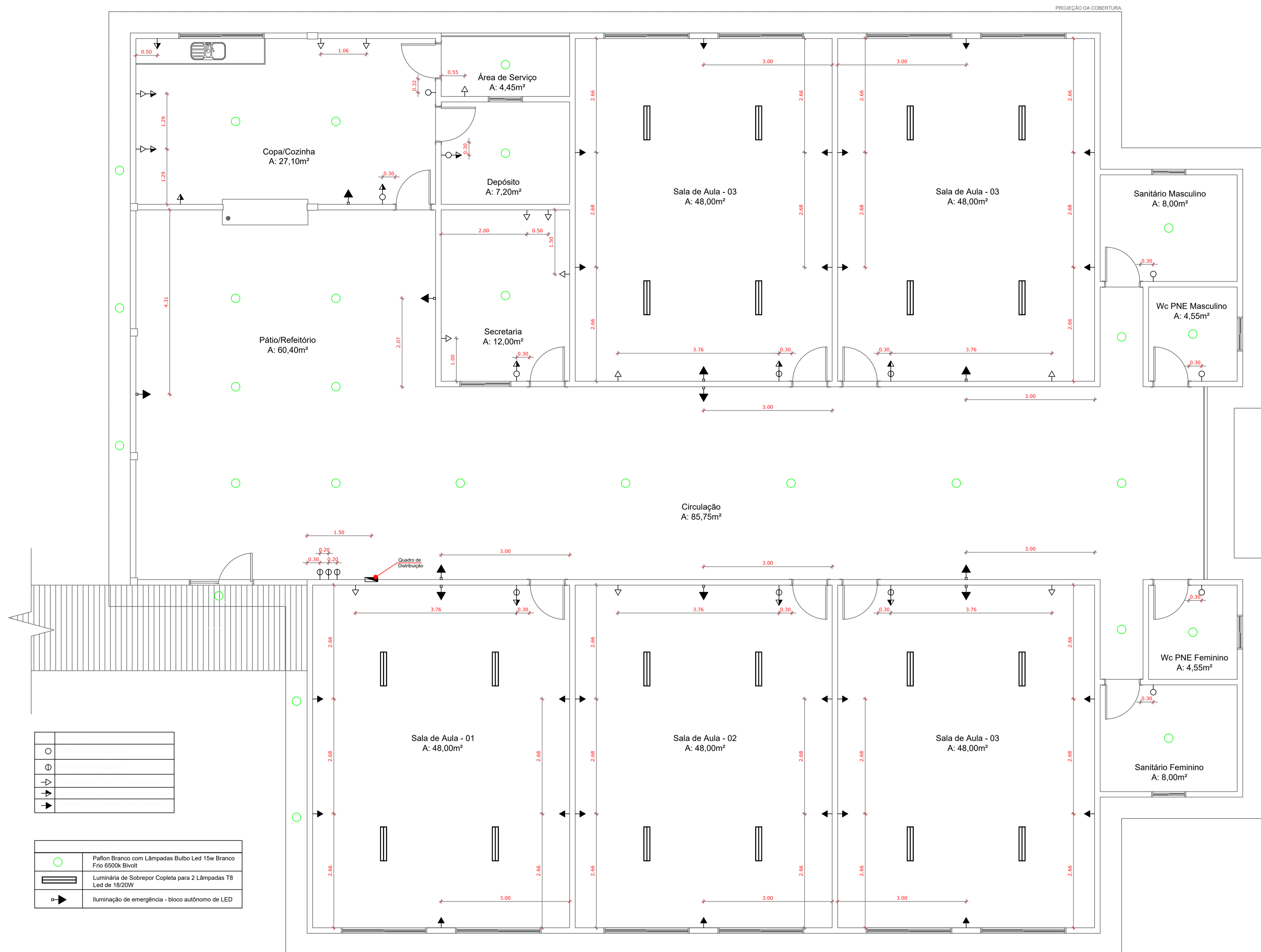
PLANTA DE ILUMINAÇÃO/ELÉTRICA.
